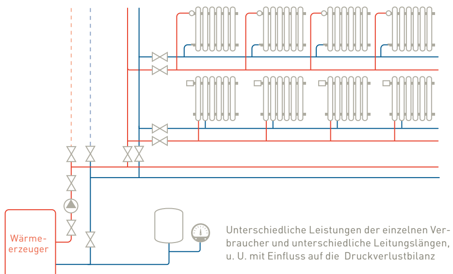
Zweirohrheizung: Typische Rohrführung in der Verteilung bei Neubauten
