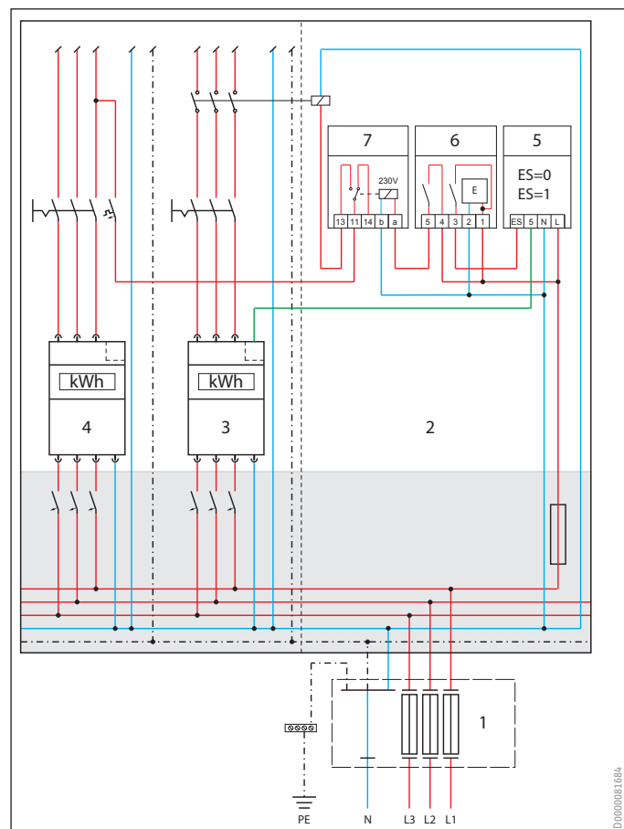
Installationsbeispiel mit Rundsteuerempfänger
