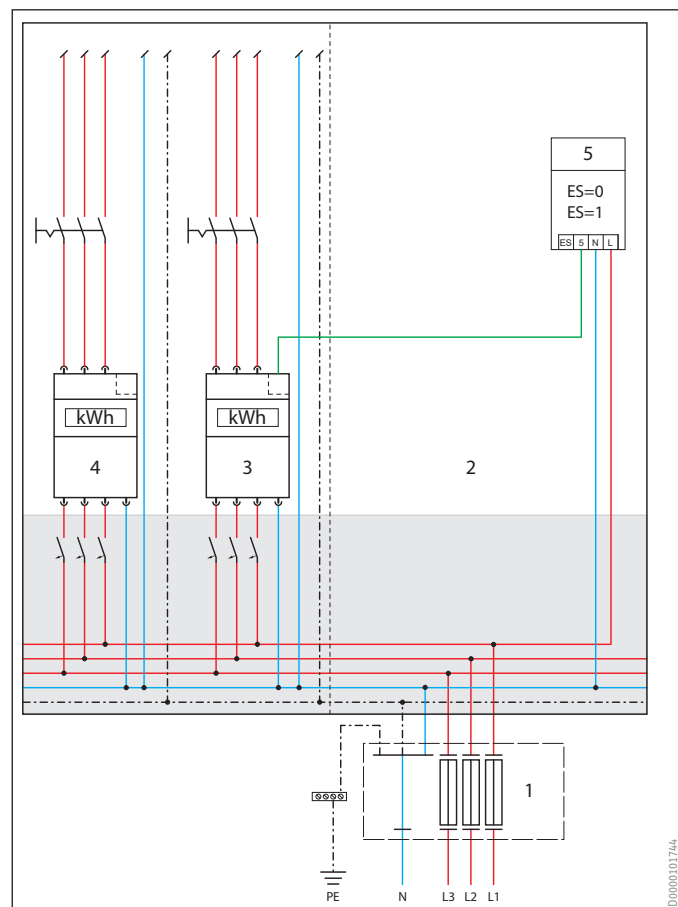
Installationsbeispiel ohne EVU-Sperre
